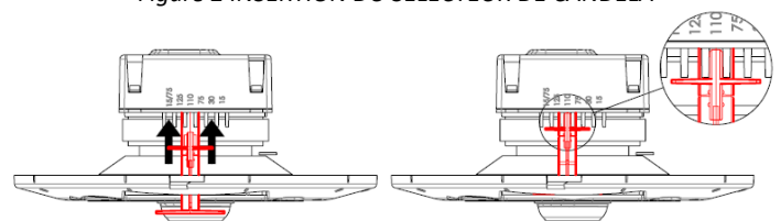
Figure 2 INSERTION DU SÉLECTEUR DE CANDELA
